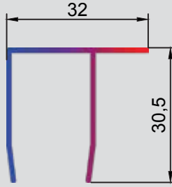
T.2802 - 0,281 kg/m
