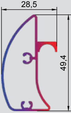
T.2801 - 0,535 kg/m
