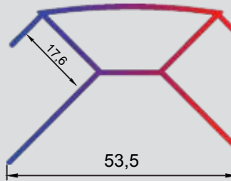
T.2809 - 0,532 kg/m
