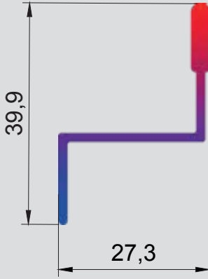
Sürme Sineklik Rayı 0,339 kg/mt
