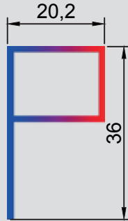
İçe Açılır Sineklik Profili 0,306 kg/mt
