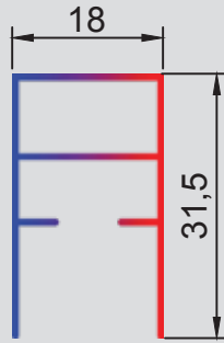
Panjur Sineklik Kasası 0,225 kg/mt
