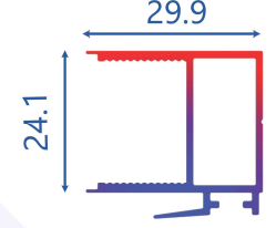
T.2356 - 0.406 KG/MT ÇEKME BAZA PROFİLİ
