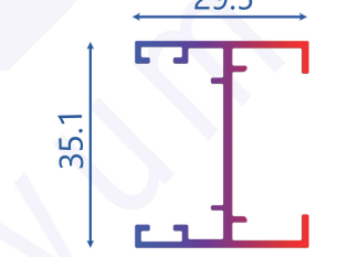
T.2359 - 0.420 KG/MT ORTA BİRLEŞİM PROFİLİ
