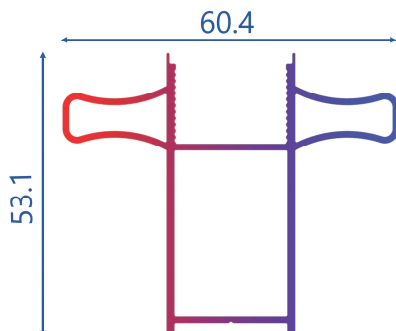
T.2358 - 0.852 KG/MT ÇİFT TARAFLI TUTAMAK
