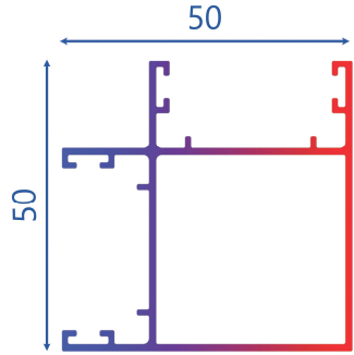
T.2360 - 0.748 KG/MT KOŞE DÖNÜŞ PROFİLİ
